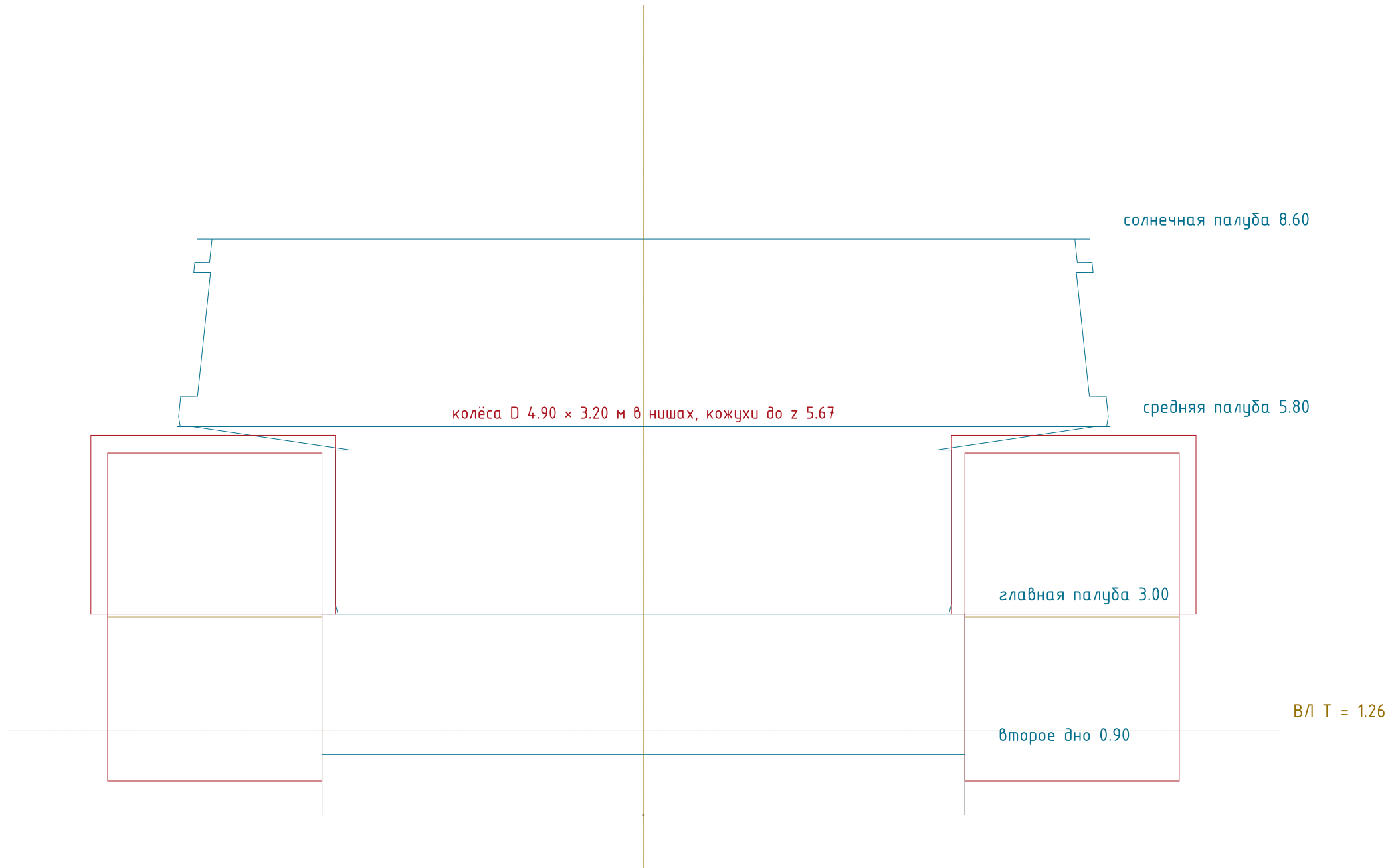
Сечение Б-Б, по оси колёс (х = 66 м)
