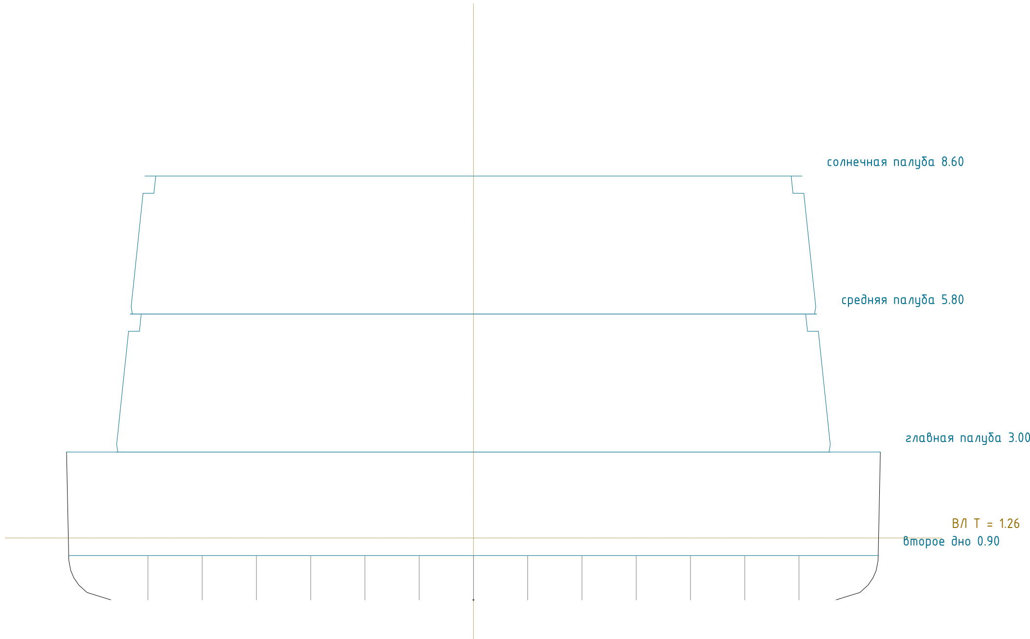
Сечение А-А, шп. 145 (х = 80 м), полная ширина
